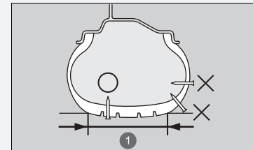
1 Kontaktfläche
