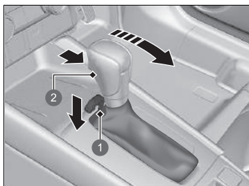
1 Schaltsperrenentriegelungsschlitz 2 Entriegelungstaste
